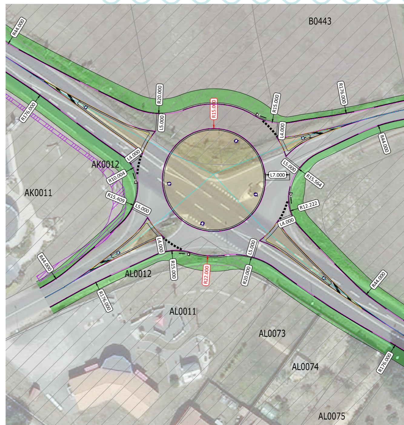
Zoom sur la réalisation d'un giratoire au carrefour des Ormeaux.
